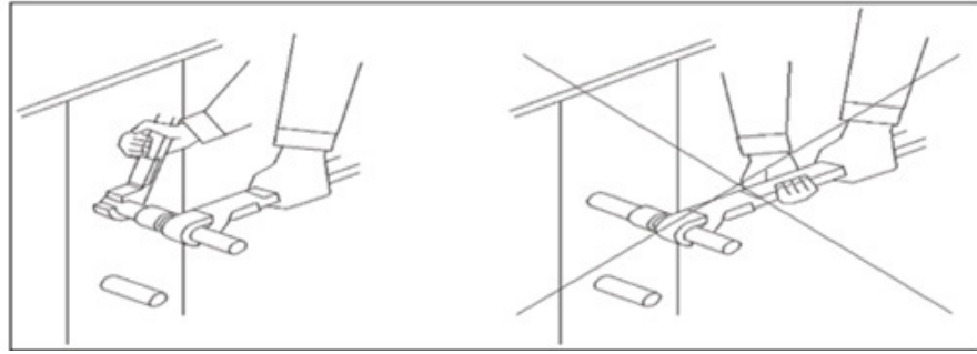
Şekil 14. Serpantin Boru Bağlantısı
